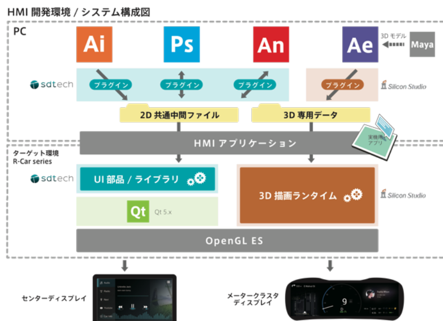
図 1: HMI 開発環境 / システム構成図
